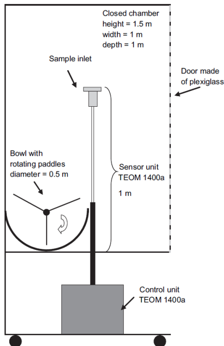
Figur 24. Exempel på apparat för laboriemätning av dammbildning hos strömmaterial vid mekanisk påverkan (Flemming m.fl. 2008)
