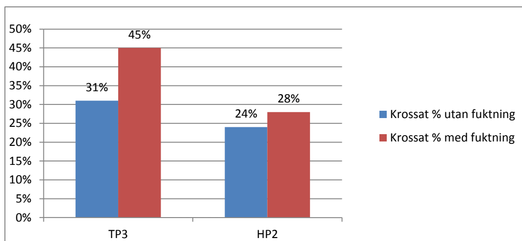
Figur 43. Sönderdelning av pellets vid belastningspulser efter uppfuktning ( 3 \times 1,69 \text{ J/cm}^2 , +10 % \text{H}_2\text{O} , efter 1 timme)
