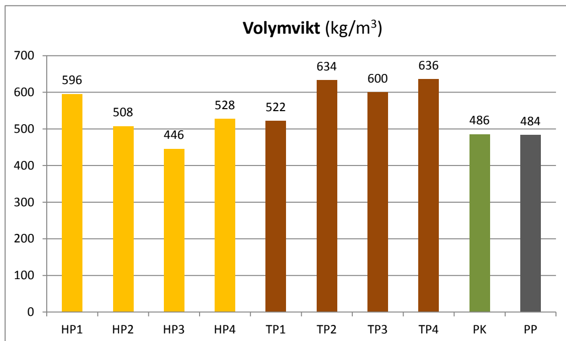
Figur 33. Volymvikt (kg/m 3 ) på olika pellets.
